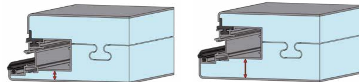
Coupe de SOLOBLOC 80.2, brevet Oméga et des différentes adaptations aux dormants
