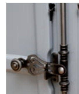
Usinage spécifique du montant du volet si fermeture par espagnolette
