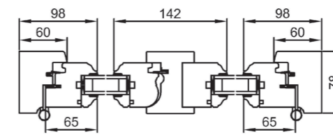
Coupe horizontale
